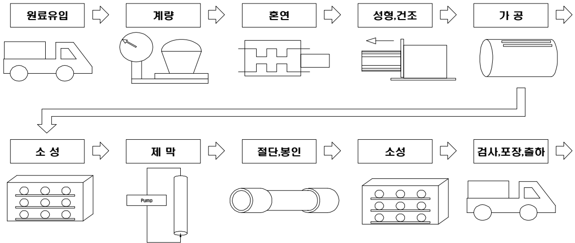
생산공정 계통도
